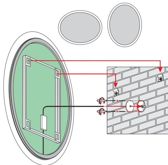
Installation position Montageposition/ Pozycja montażu
