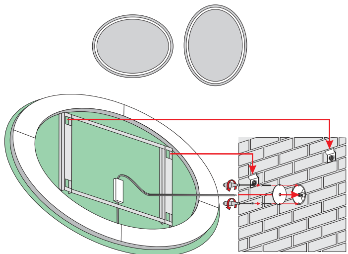
Installation position Montageposition/ Pozycja montażu
