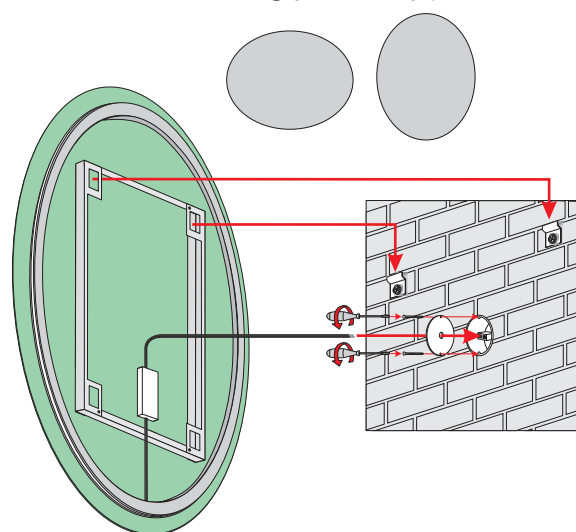
Installation position Montageposition/ Pozycja montażu
